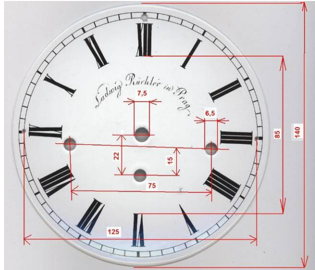
Ciferník smalt č. 2 – se signaturou
