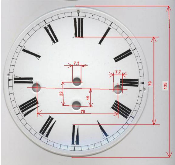
Ciferník smalt č. 1 – bez signatury
